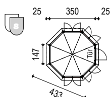
Grunewald Typ 1 8-Eck-Pavillon, geschlossen
