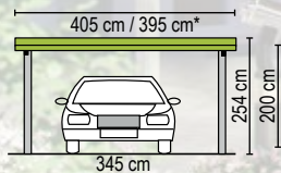
Modell „Flensburg L (F), Natur“
