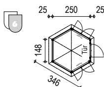
Dahlem Typ 1 6-Eck-Pavillon, geschlossen
