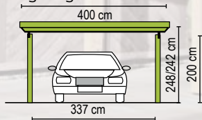
Modell „City -Carport 1“
