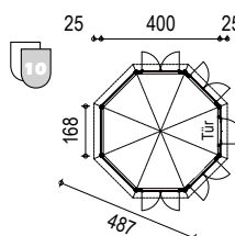
Grunewald Typ 2 8-Eck-Pavillon, geschlossen
